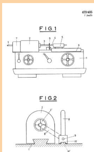
CH473635A Tour révolver
