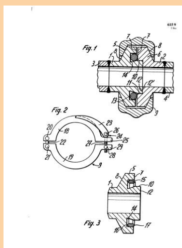
CH615988A5 Raccord métallique
